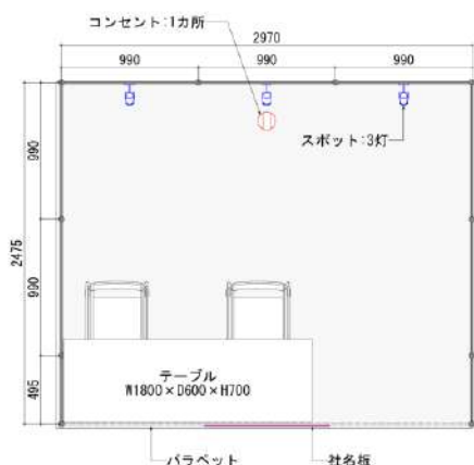
※平面図
