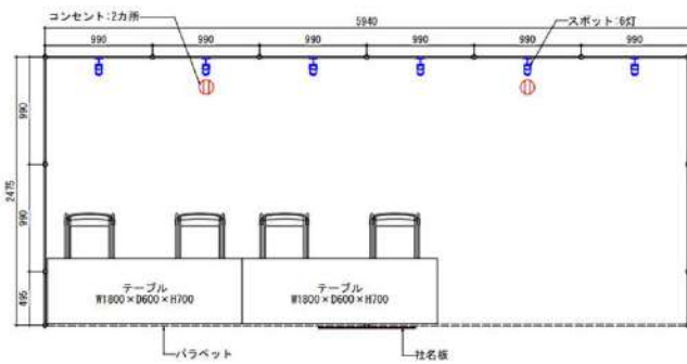
※平面図
